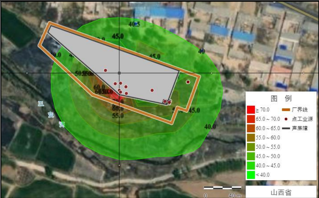
图4-2 本项目昼间噪声贡献等值线图
