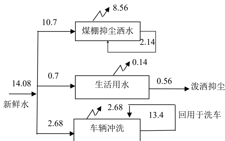
图 2-1 项目用排水平衡图 ( \text{m}^3/\text{d} )
