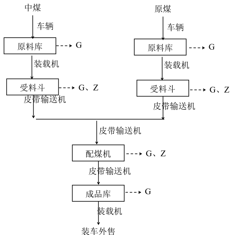
图 2-3 运营期工艺流程及产污节点图
